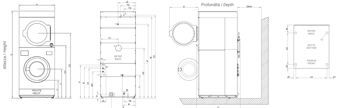
Pos. 1 - Acqua fredda lavatrice / Washing machine cold water Ø 3/4"; Pos. 2 - Acqua calda lavatrice / Washing machine hot water Ø 3/4"; Pos. 3 - Vapore diretto lavatrice (macchine vapore) / Washing machine direct steam (only steam heated machine); Pos. 4 - Scarico acqua lavatrice / Washing machine water drain Ø 50 mm; Pos. 5 - Sfiato lavatrice / Washing machine Ø 50 mm; Pos. 6 - Scarico aria umida e fumi (essiccatoio) / Humid air and smoke exit (Dryer) TDM 1111 Ø 100 mm, TDM 1818 Ø 150 mm; Pos. 7 - Alimentazione elettrica (presa unica) / Electrical power supply; Pos. 8 - Scarico condensa vapore essiccatoio (macchine vapore) / Dryer input steam (only steam heated machine) Ø 3/4" - 1"; Pos. 9 - Ingresso vapore essiccatoio (macchine vapore) / Dryer input steam (only steam heated machine) Ø 3/4" - 1"; Pos. 10 - Scarico condensa lavatrice (macchine vapore diretto) / Washing machine steam drain (only direct steam heated machine); Pos. 11 - Connessione GAS (solo essiccatoi a GAS) / GAS supply (only GAS heated dryers) Ø 3/4"; Pos. 12 - 4 Piedini macchina "M10" / 4 "M10" feet - 100 mm = 3.93 inch. - fattore di conversione 1 / 25,4 \ factor conversion 1 / 25,4
